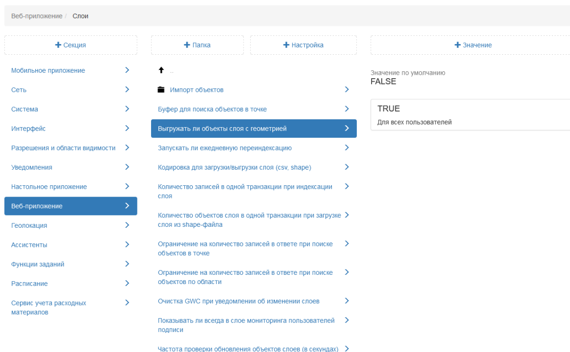
Рис. 2.285: Настройка выгрузки слоя с геометрией объектов
