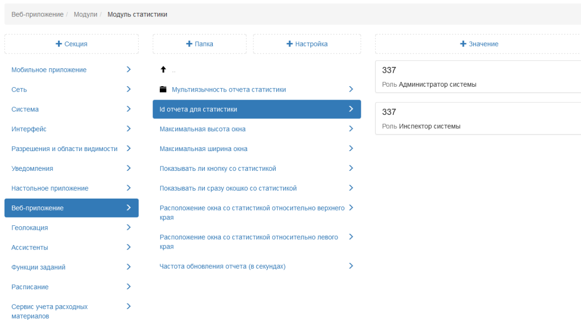
Рис. 2.268: Указание отчета для модуля статистики
