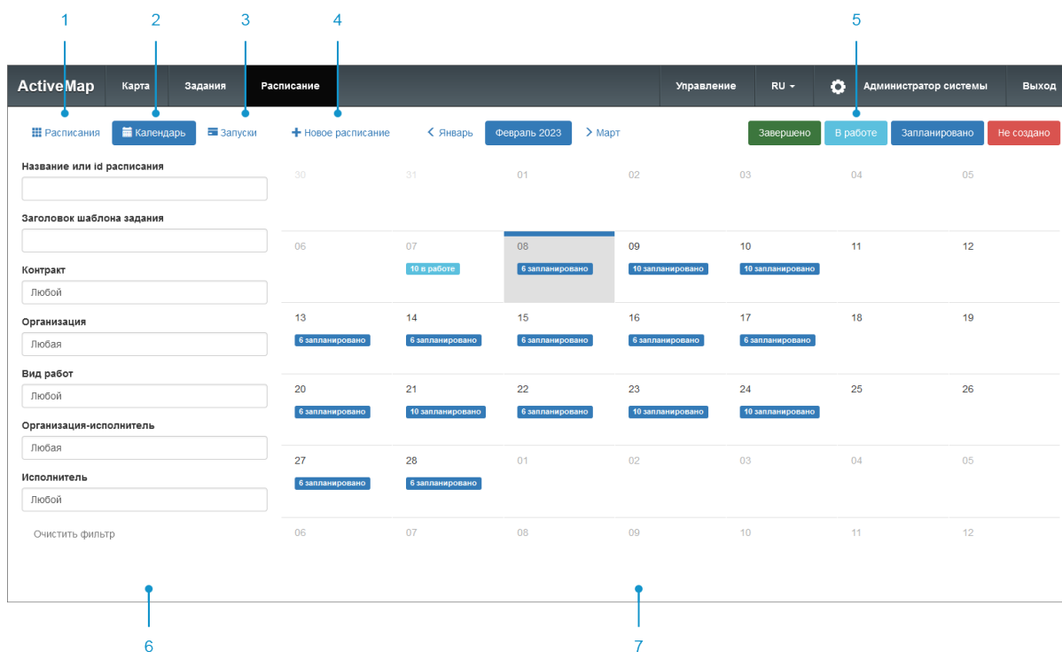
Рис. 2.27: Окно расписаний с календарем
