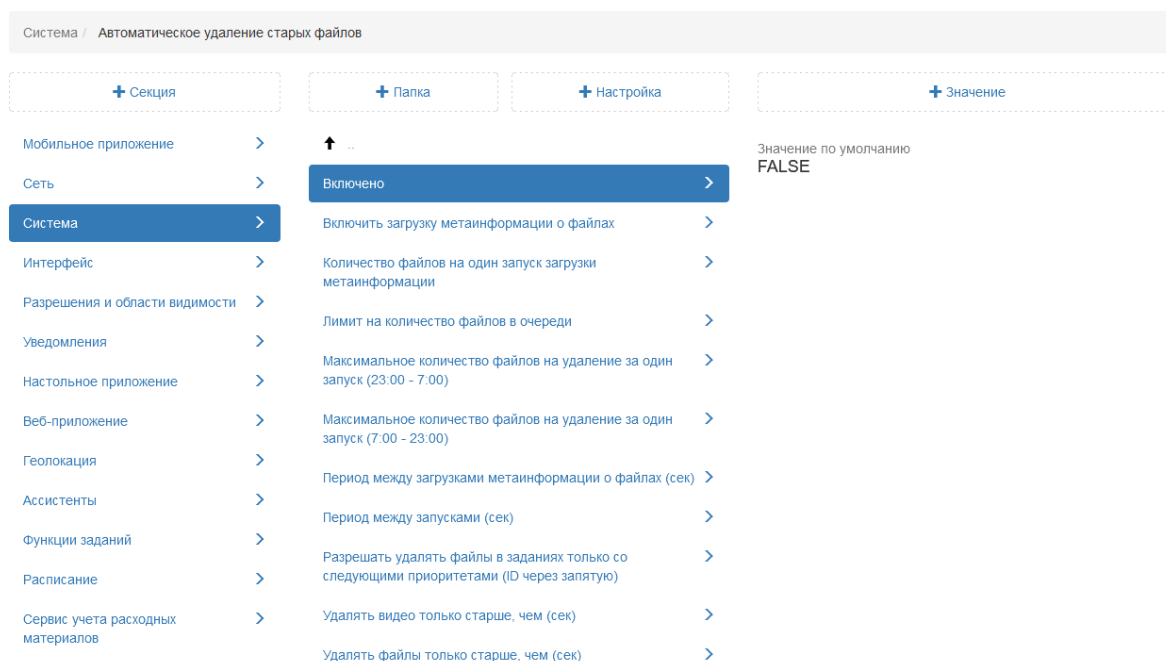
Рис. 2.204: Автоматическое удаление старых файлов
